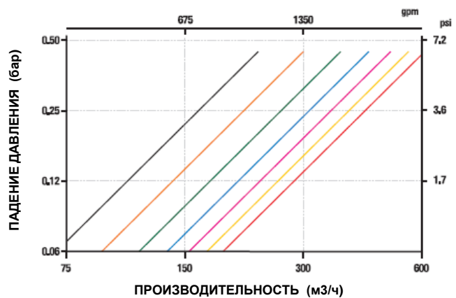
ПАДЕНИЕ ДАВЛЕНИЯ В СИСТЕМЕ AZUD HELIX AUTOMATIC 130 мкм
